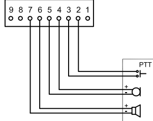
Terminal J8
